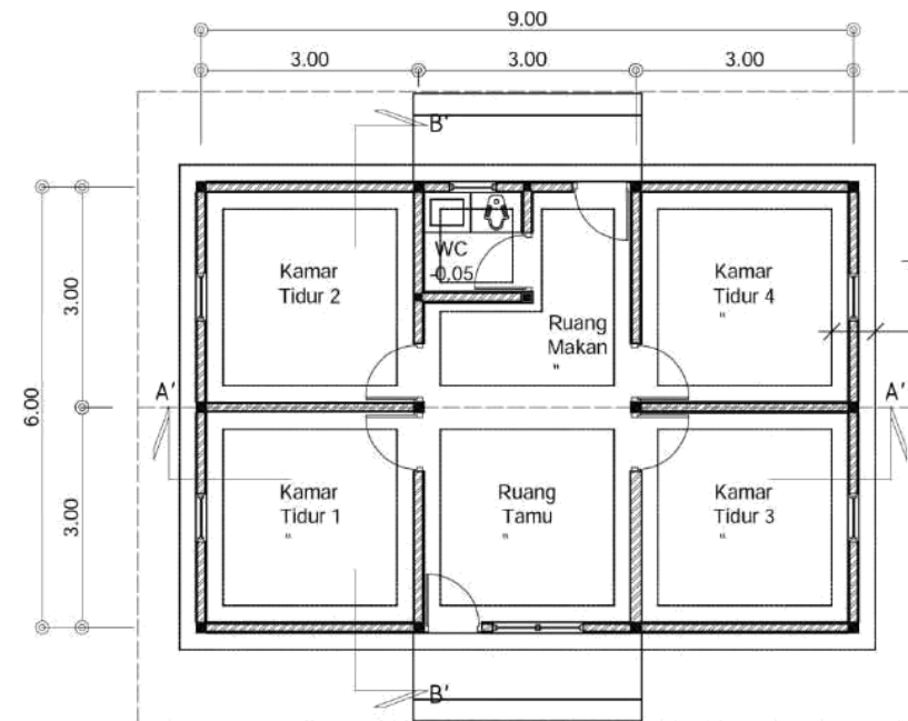
DENAH SKALA 1 : 100
