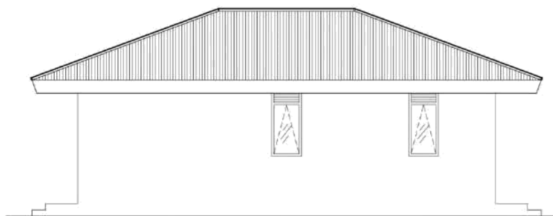
TAMPAK SAMPING KIRI SKALA 1 : 100
