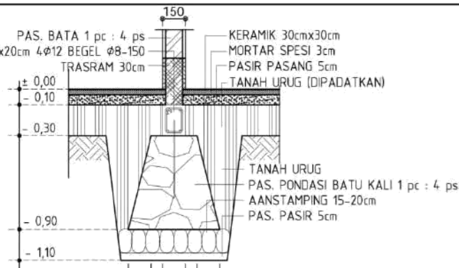
FONDASI SKALA 1 : 30
