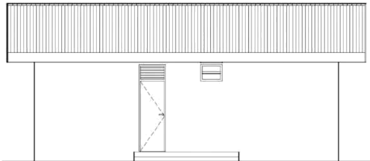
TAMPAK BELAKANG SKALA 1 : 100
